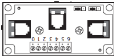
Bild: Optionale T- Abzweigung für Bedienteil Kabel
